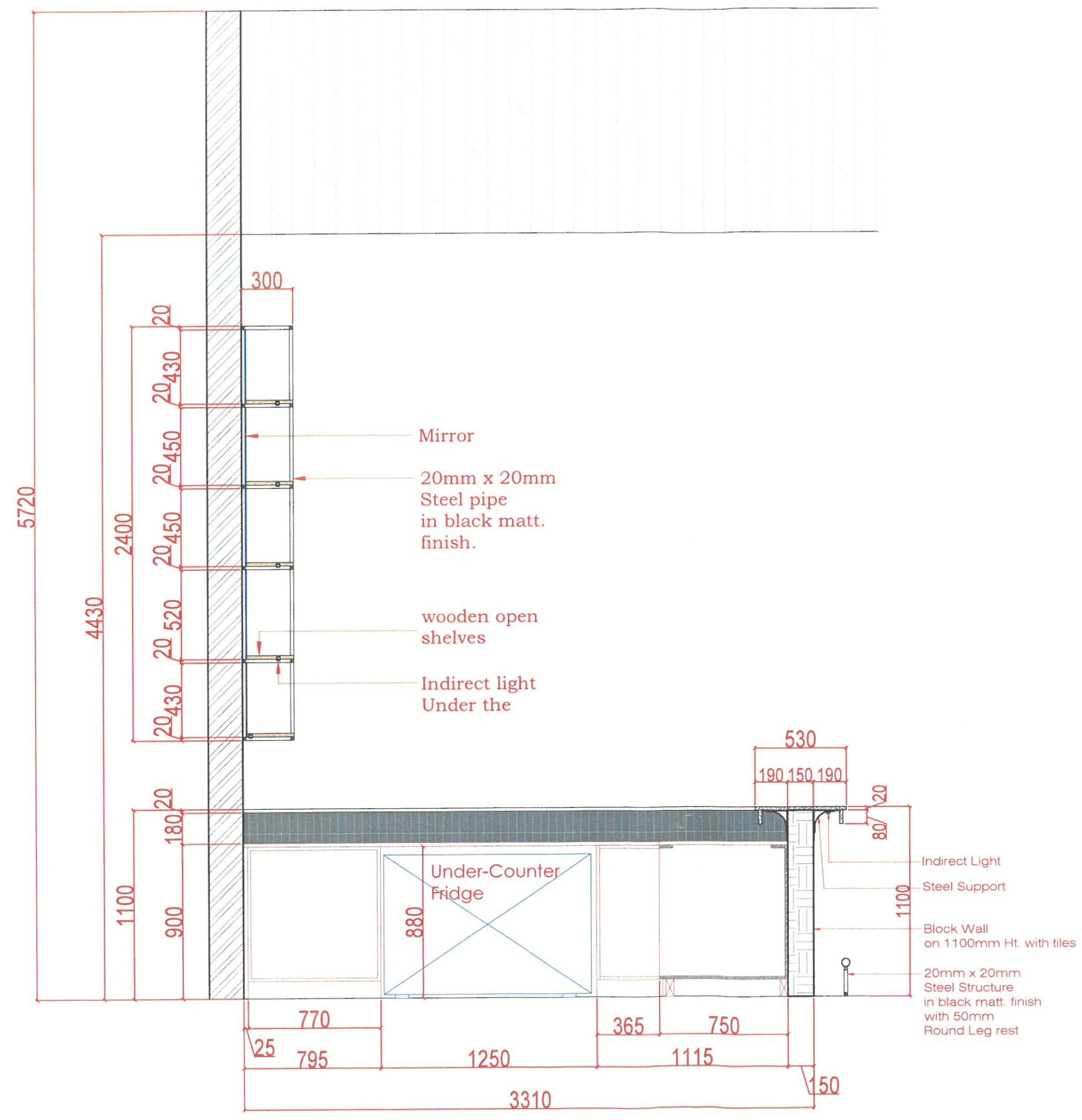
Elevation - D
